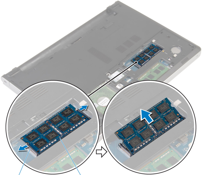
1 Ganchos de fijación (2)
